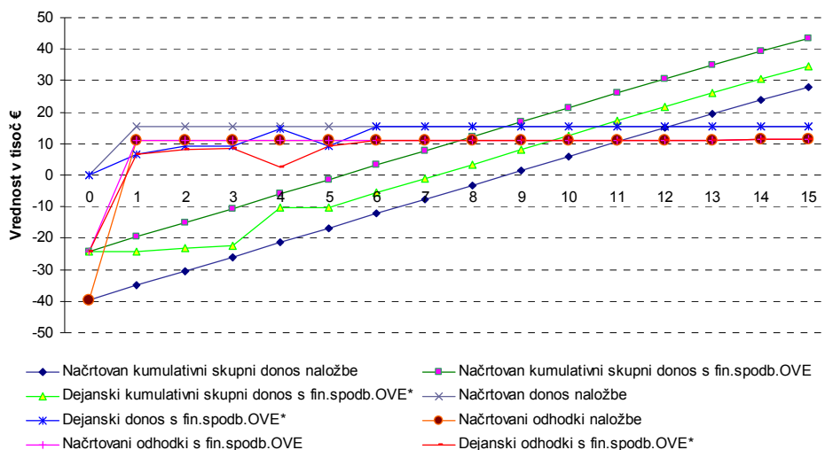
Slika 4: Realni denarni tok in doba vračanja naložb Toplotne črpalke Opomba: *dejansko stanje velja za obdobje 2005-2009, nadalje so načrtovane vrednosti
