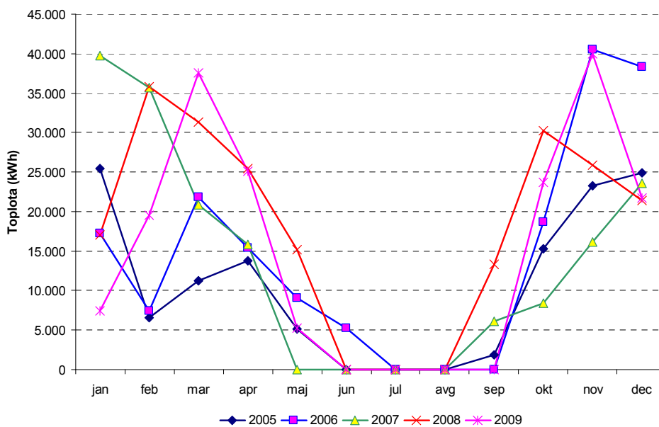
Slika 2: Proizvodnja toplote (kWh)
